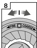
8 Déplacez la meule supérieure réglable, 1 chiffre, mouture plus grossière (coarse) ou plus fine (fine)
